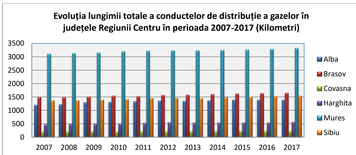
Figura 3.2.9 Sursa datelor: Institutul Național de Statistică
