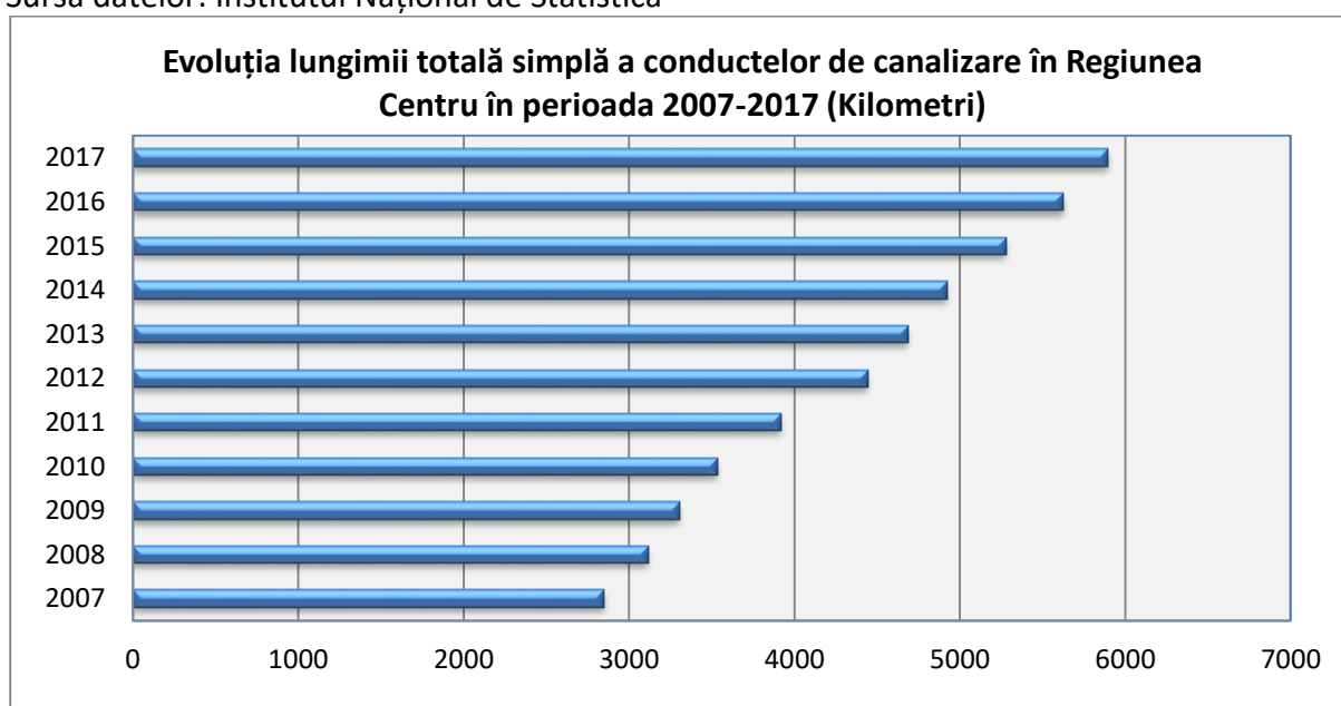
Figura 3.2.6 Sursa datelor: Institutul Național de Statistică
