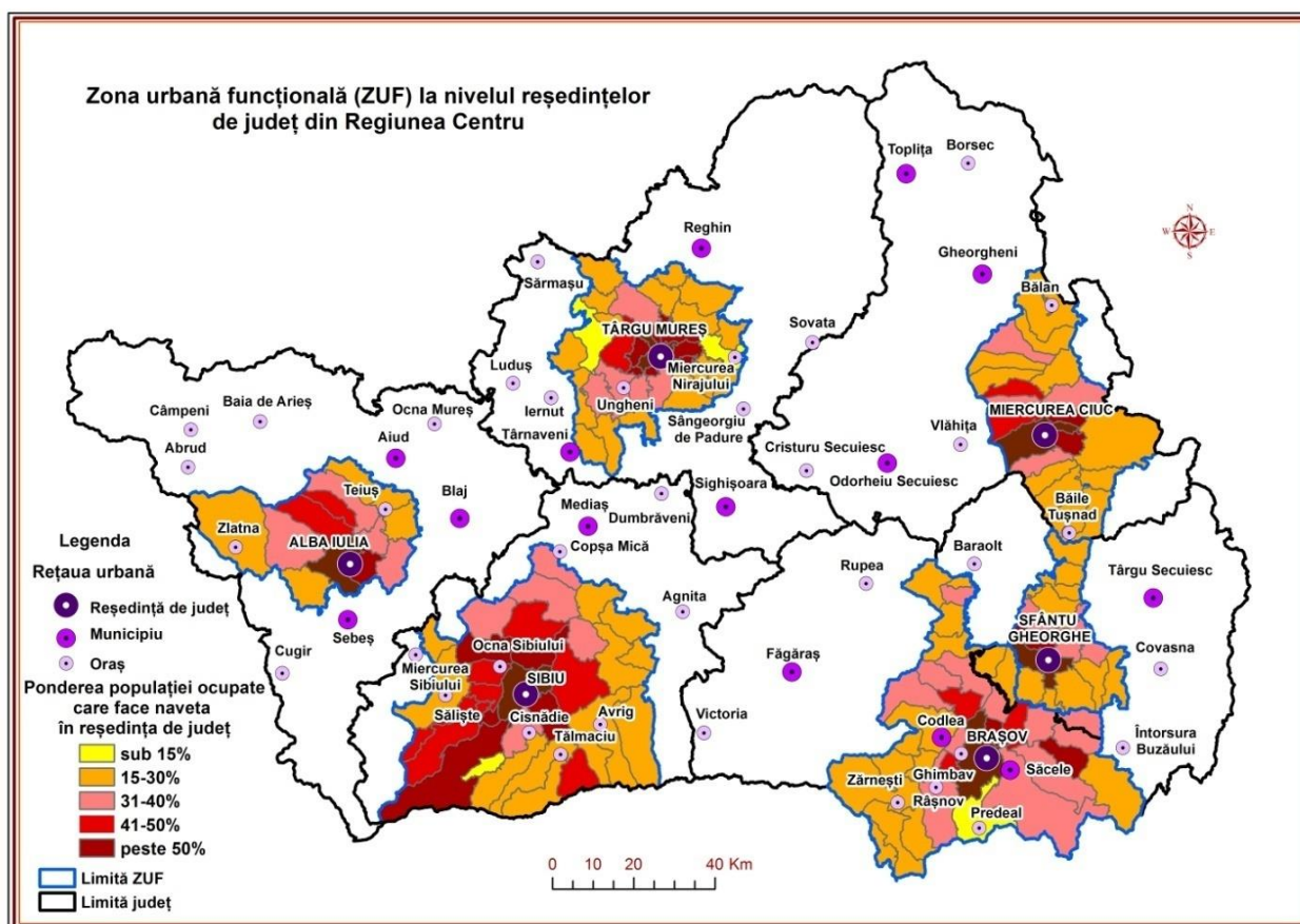
Figura 1.6 Localizarea geografică a zonelor urbane funcționale la nivelul reședințelor de județ din Regiunea Centru (Harta: ADR Centru, Sursa datelor: Banca Mondială 4 , 2017)
