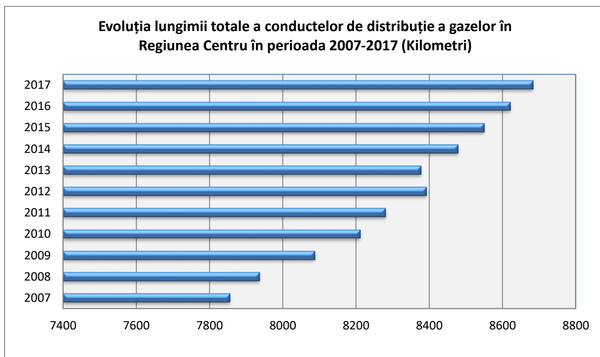
Figura 3.2.8 Sursa datelor: Institutul Național de Statistică
